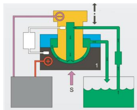
Princip obrábění
